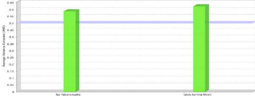
Grafik 1. AVE Değerleri
