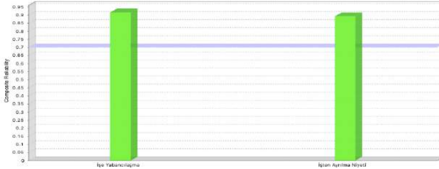
Grafik 2. Birleşik Güvenirlilik (CR) Değerleri
