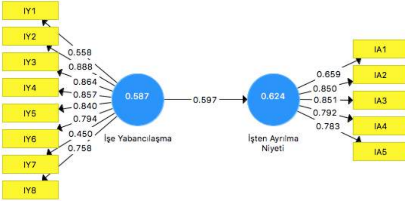
Şekil 2. Hizmet Sektörü Kadın Çalışanlarda İşe Yabancılaşmanın İşten Ayrılma Niyeti Üzerindeki Etkisi Yol Analizi
