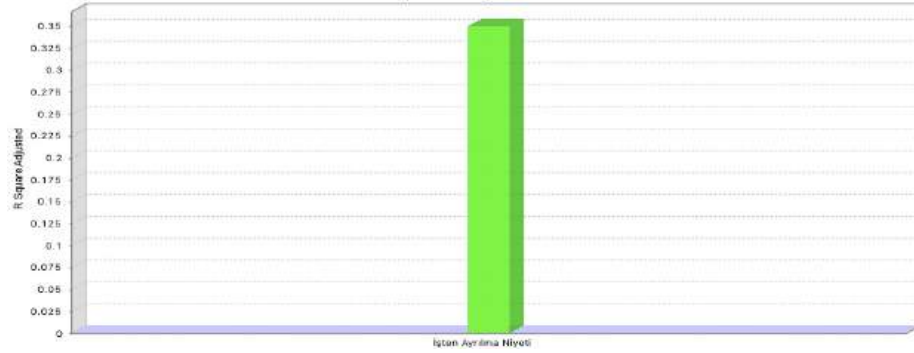
Grafik 3. R^2 Değerleri
